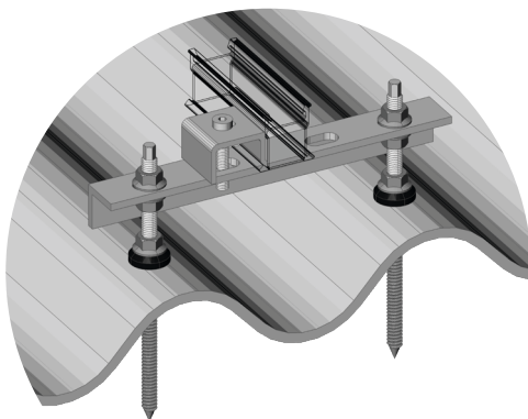
EINFACHE MONTAGE AUF WELLETERNIT
