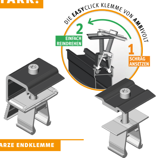
SCHWARZE MITTELKLEMME
